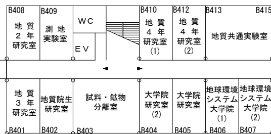
理学部B棟 4階平面図
