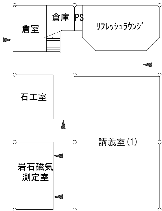
理学部講義棟 1階平面図
