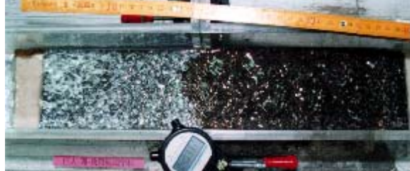
図3 幅10cmの水路で、植生の有る無しによる土砂の運ばれ方の違いを観察。ビニル紐で草を植えると、水流で倒れて布団を敷いたよう。その上を一番大きい石を先頭に列を作って土砂がコロコロと運ばれる。砂礫だけでは粒同士がかみ合って動きが遅い。
