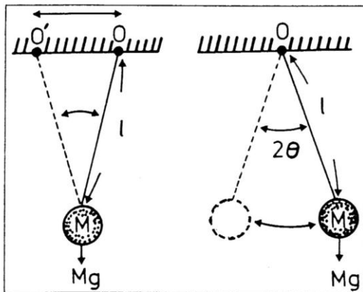
図1 ふりこ げんり 振子の原理
