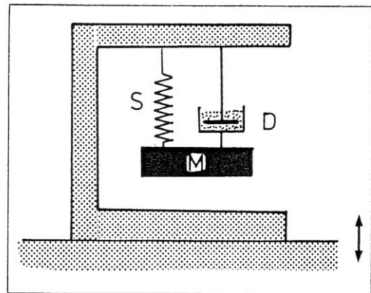
図2 じやうげどうじしんけい げんり 上下動地震計の原理
