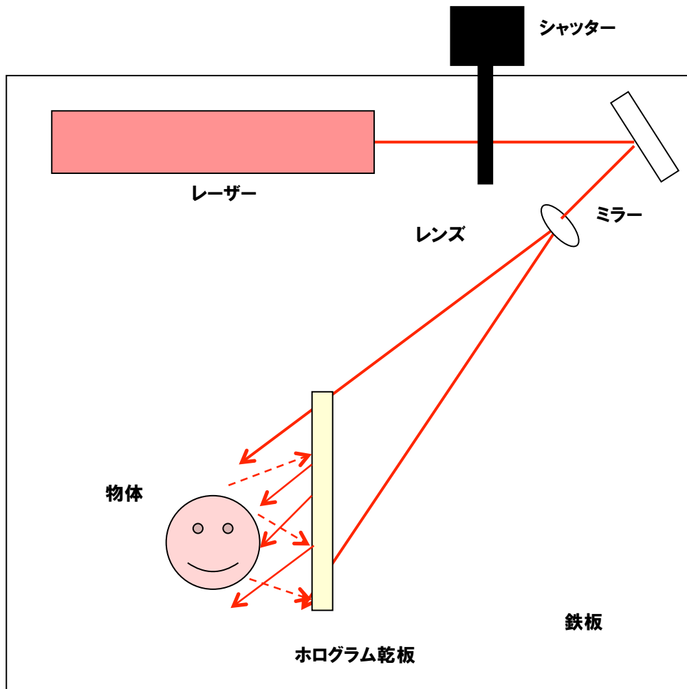
デニシユクホログラムの光学系
